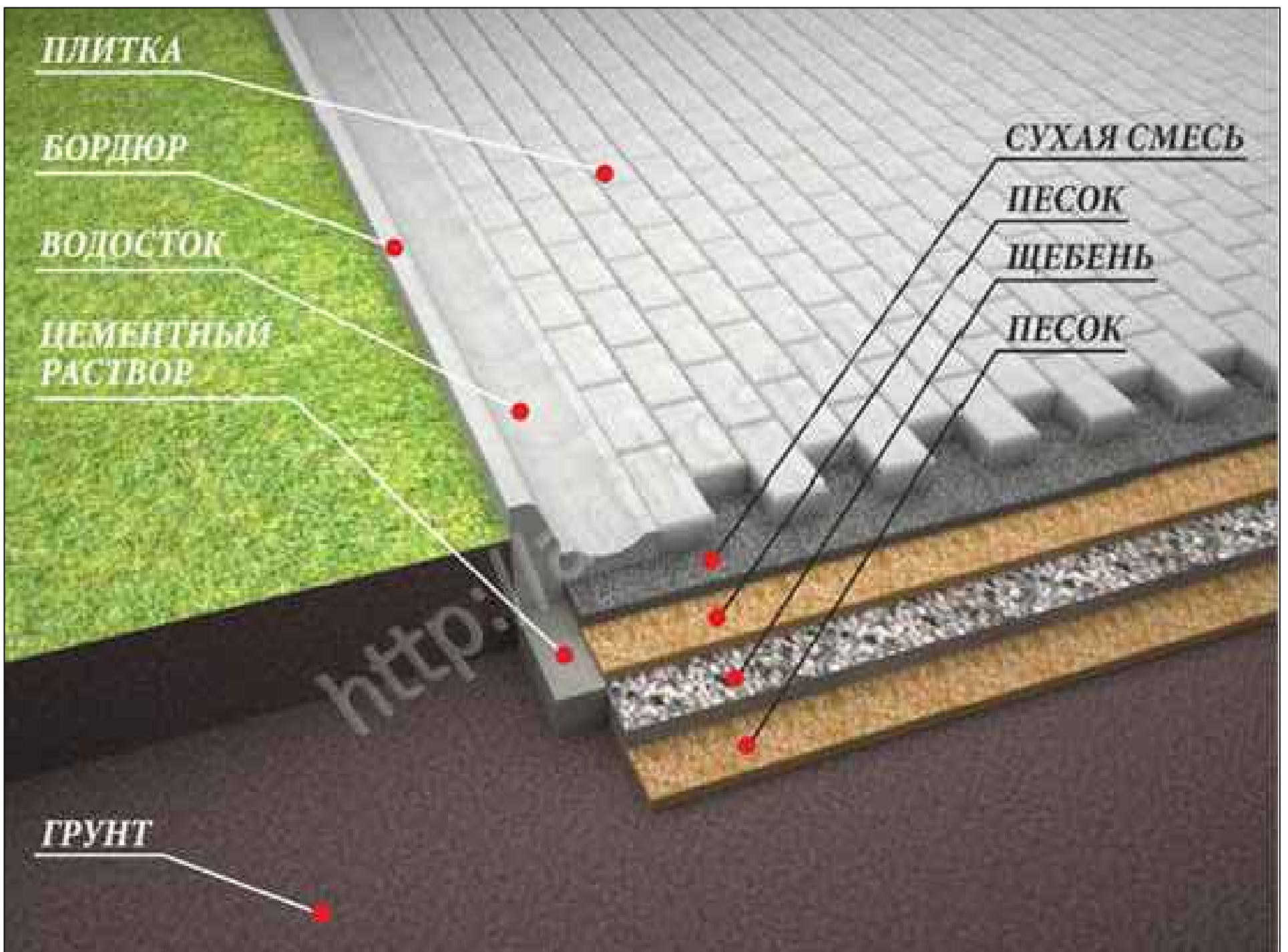
Схема влаштування дорожнього покриття з бруківки
